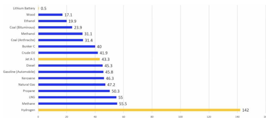
Energía específica (MJ/kg) de diferentes combustibles y baterías [IATA]
