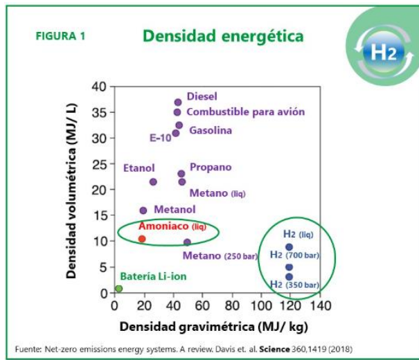
Energía específica (o 'Densidad gravimétrica) vs. Densidad energética (o 'Densidad volumétrica) de diferentes combustibles aeronáuticos
