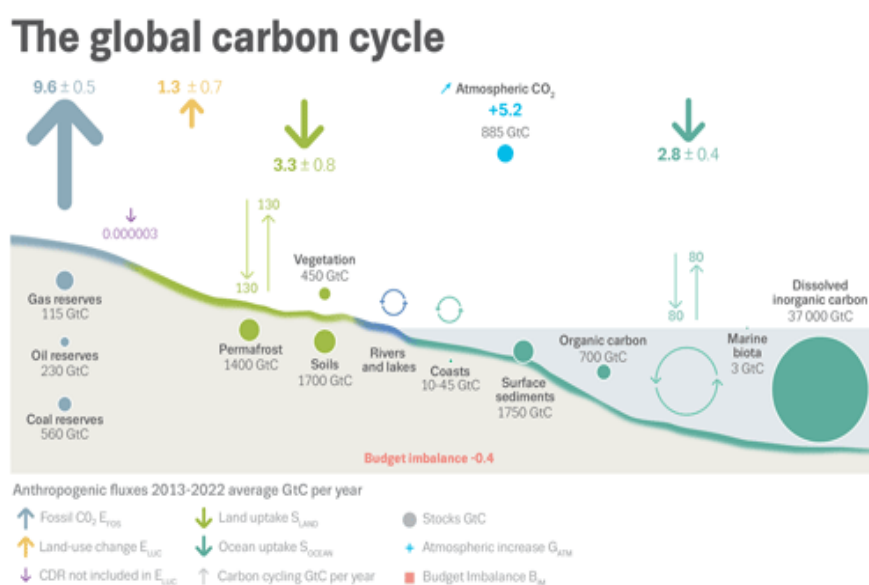
Representación esquemática de la perturbación general del ciclo global del carbono causada por actividades antropogénicas, promediada a nivel mundial para la década 2013-20227
