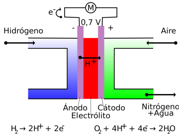
Funcionamiento básico de una pila de hidrógeno 125
